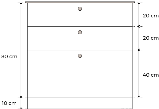
Modelo C500 Altura de encimera con armazón 80 cm
